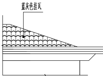
变更前局部立面图
