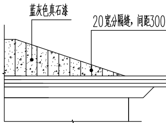
变更后局部立面图
